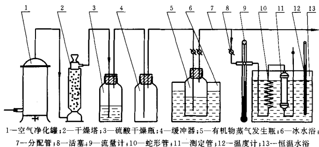
图1 吸附率测定装置及其流程示意图
